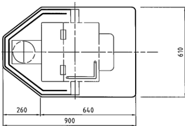
各部寸法
