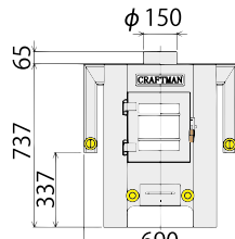
正面図
