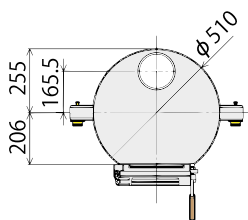
上面図
